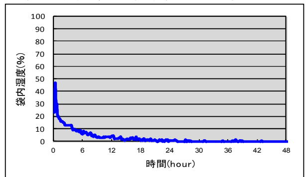
袋内湿度挙動例 (空袋 絶乾タイプの場合)
