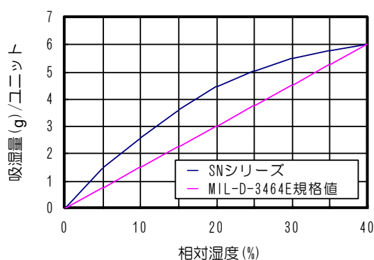
吸着等温線 (25℃)
