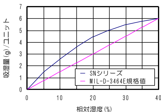
吸着等温線 (25℃)
